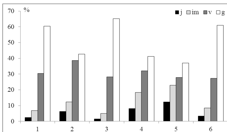
Рис. Возрастные спектры ценопопуляций Neotinea ustulata . j — ювенильные, im — имматурные, v — виргинильные, g — генеративные растения. По оси абсцисс — номера ценопопуляций (1–6); по оси ординат — доля возрастной группы в спектре, %.
