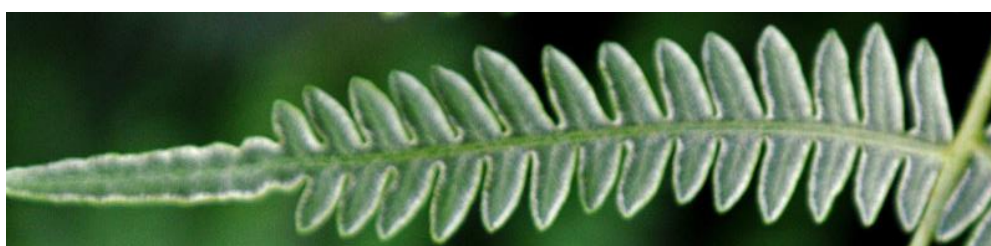
Рис. 4. Сегмент вайи Pteridium pinetorum . Fig 4. Vaya segment of Pteridium pinetorum .
